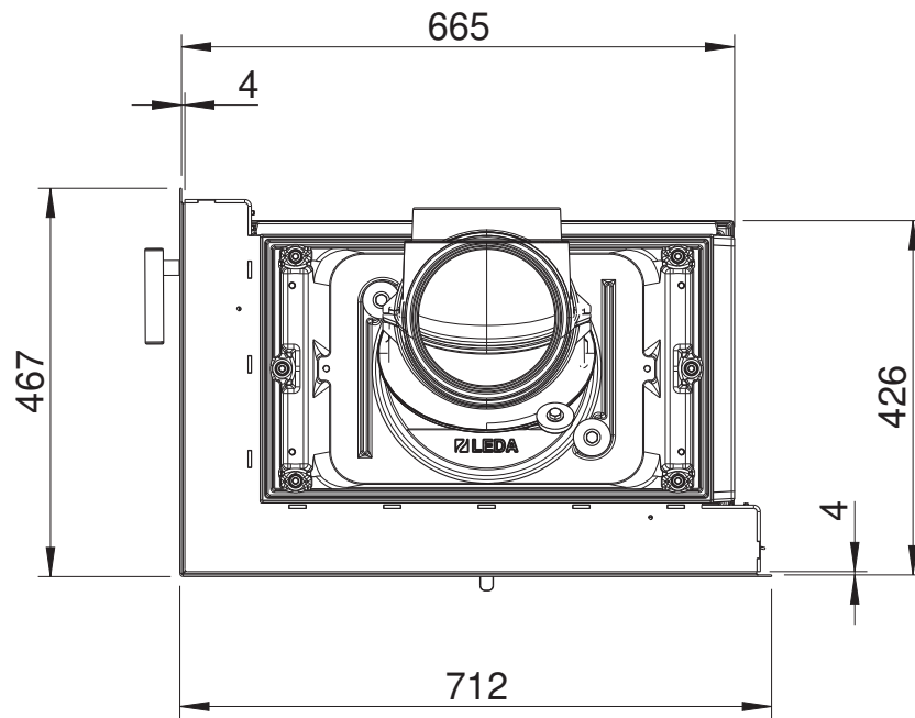
Blendrahmen am FINA ES L/ FINA plus ES L (Draufsicht, Massstab 1:10)
