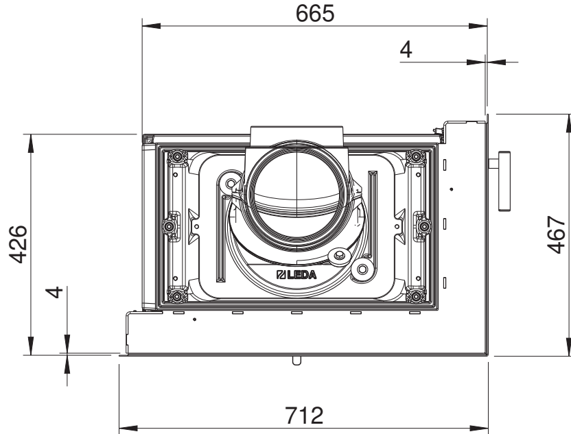
Blendrahmen am FINA ES R/ FINA plus ES R (Draufsicht, Massstab 1:10)
