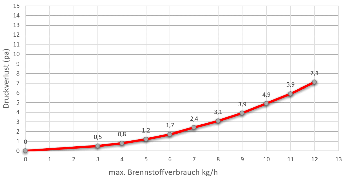
Druckverlustdiagramm GT 44/50
